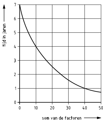
Figuur 1. Periodieke controle (figuur K.1 uit 'bijlage K' van NEN 3140:2011)
